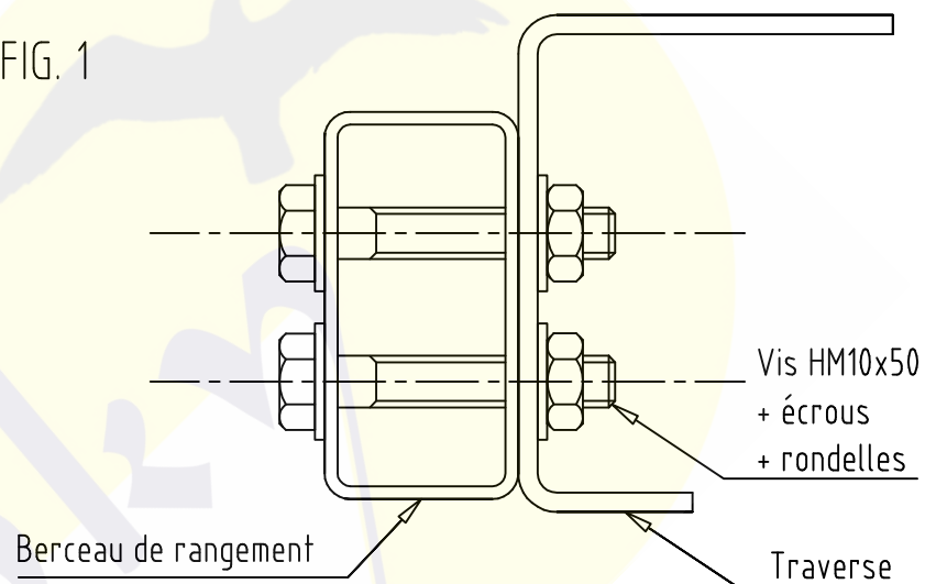
Détail fixation berceau
